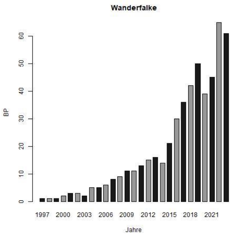
Abb. 1: Bestandsentwicklung des Wanderfalken in Mecklenburg-Vorpommern im Zeitraum 1997-2023.
